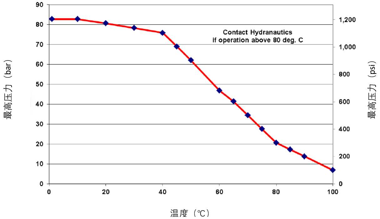
最高压力 Vs. 温度曲线图
