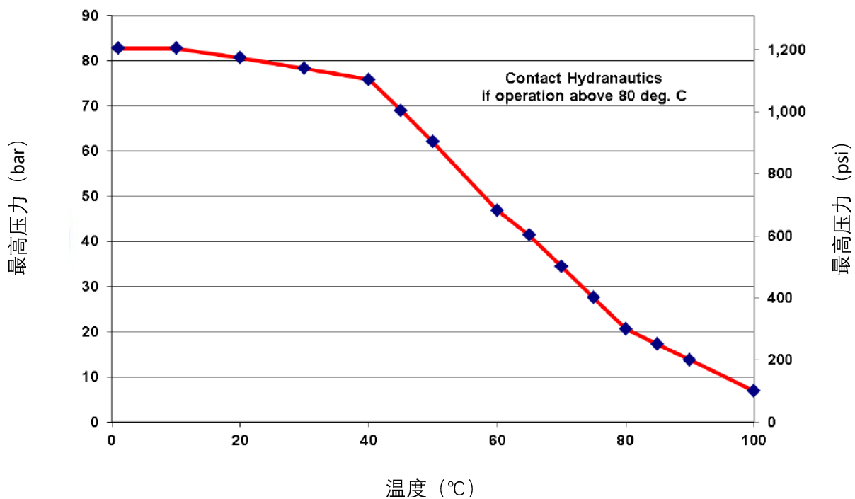
最高压力 Vs. 温度曲线图
