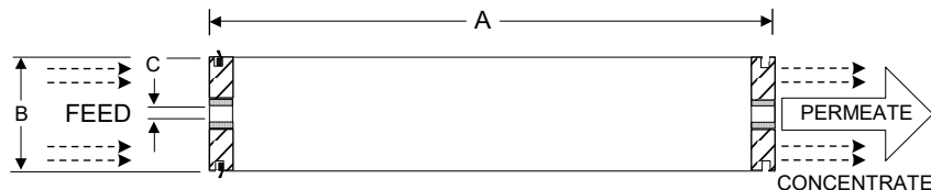
膜元件尺寸**
