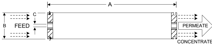
膜元件尺寸**
